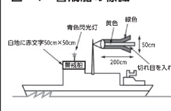
図-4 警戒船の標識
