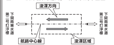
図-7 浚渫船「海翔丸」の作業状況側面図
