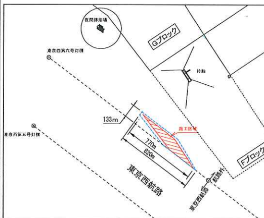
浚渫工 施工位置図
