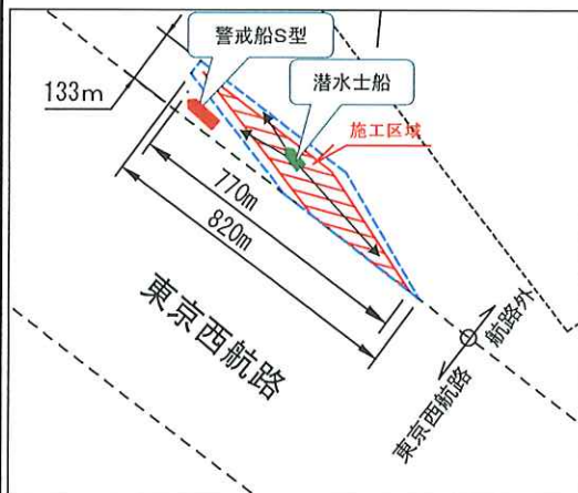
潜水探査 作業船配置図
