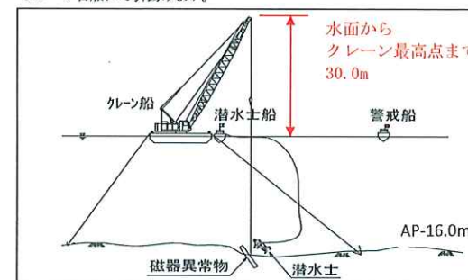
潜水探査 作業状況図
