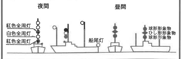
図-8 浅渚船「海翔丸」の灯火及び形象物
