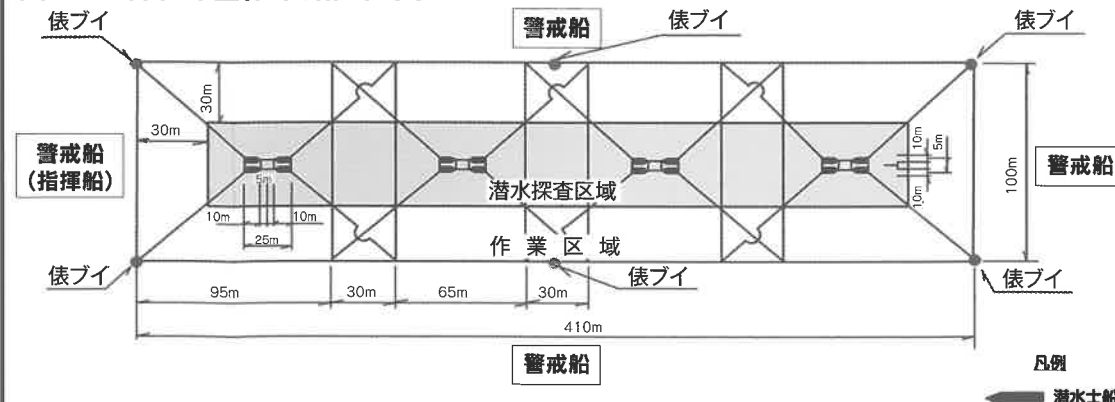
圖-2 潜水探查作業船配置図
